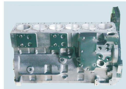
Short Block 6C/ISL TPEC-6C/ISL短缸体
