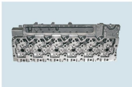
Cylinder Head QSL8.9L TPEC-QSL8.9缸盖
