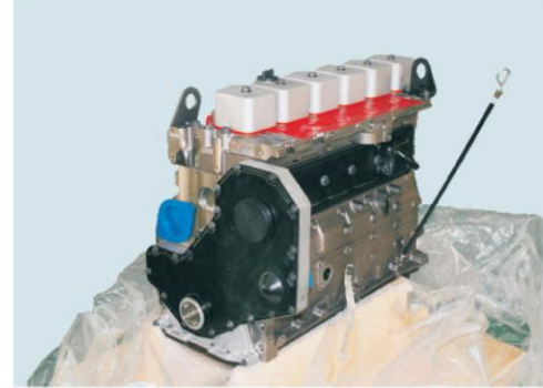
Long Block 6BT5.9 TPEC-6BT5.9长缸体
