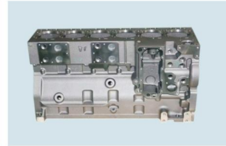
Cyl Block ISLe 8.9 New Type TPEC-ISLe新款缸体 5662123
