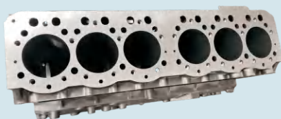
Cylinder Block S6K/3066 TPEC-S6K/3066缸体
