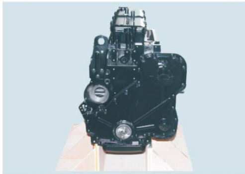
Long Block ISL 8.9 TPEC-ISL 8.9长缸体
