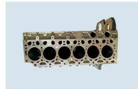
Cylinder Block D6E TPEC-D6E缸体
