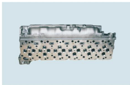
Cylinder Head ISDe/QSB6.7L TPEC-ISDe/QSB6.7缸盖 3977225
