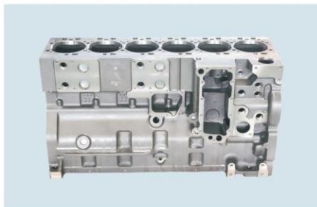
Cyl Block 6LTA8.9 4928830 TPEC-6LTA8.9缸体 4928830
