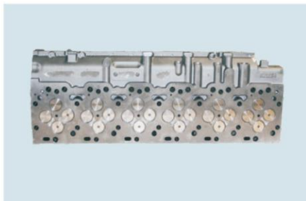
Cylinder Head Assy QSL8.9L TPEC-QSL8.9缸盖总成
